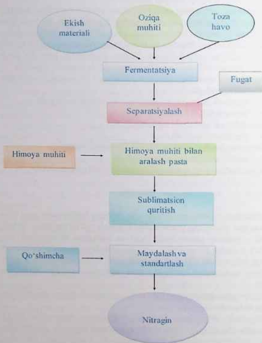
1-rasm. Nitragin ishlab chiqarishning texnologik chizmasi
