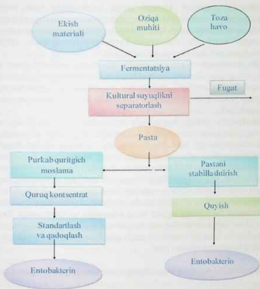
8-rasm. Entobakterin ishlab chiqarish texnologiyasining chizmas
