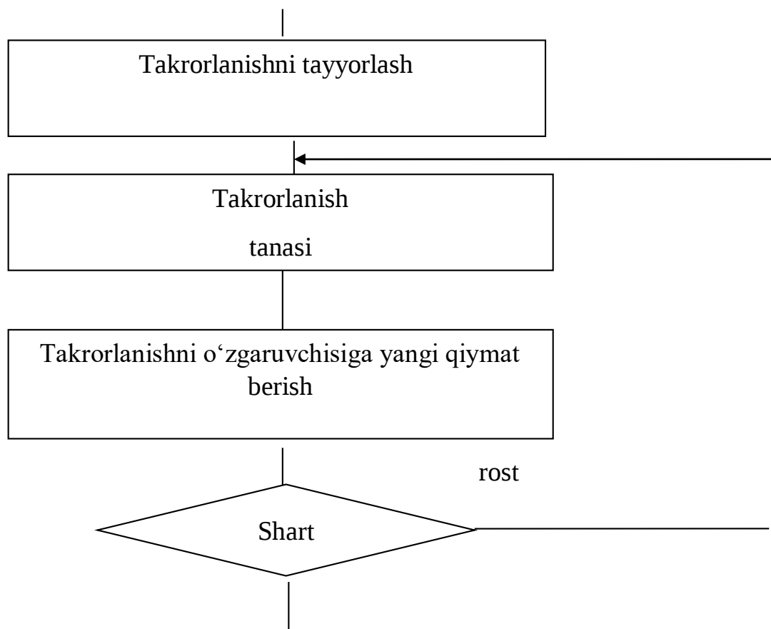
12.6-rasm. Sharti keyin tekshiriladigan takrorlanish algoritmining blok sxemasi
