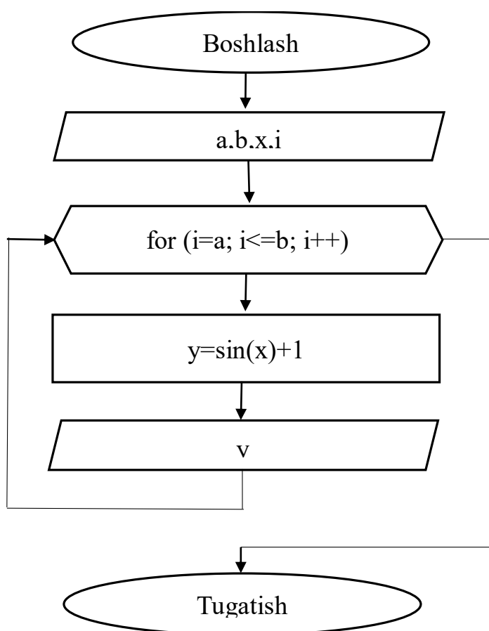
12.13-rasm. Dastur blok sxemasi
