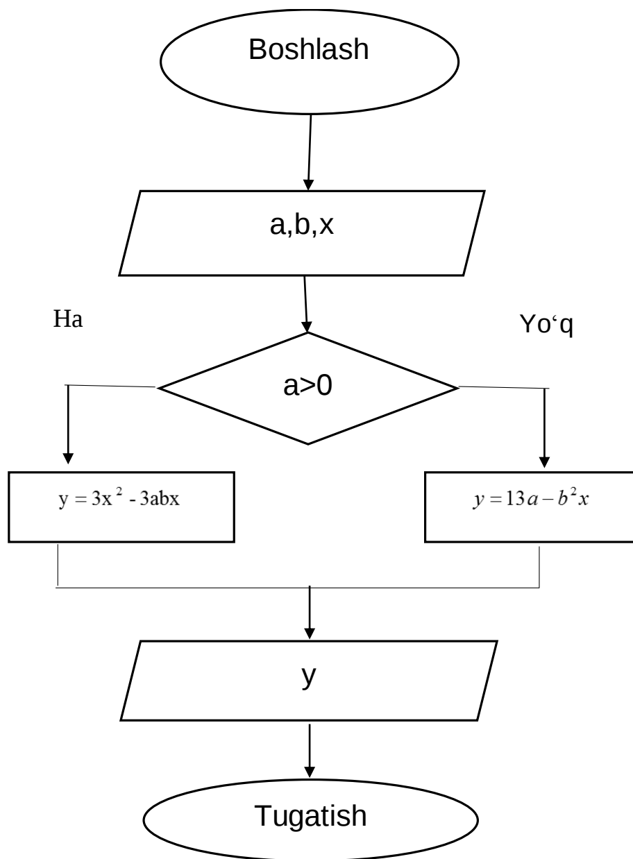
11.2-rasm. Dastur blok sxemasi
