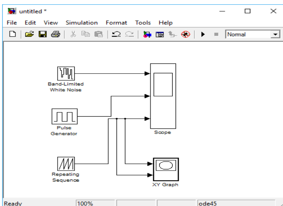
5.8-rasm. Modelning sxemasi
