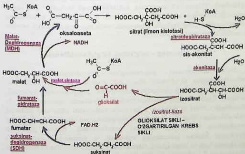
45-rasm. Gliksolat siklining sxemasi(V.V. Polevoy bo'yicha).
