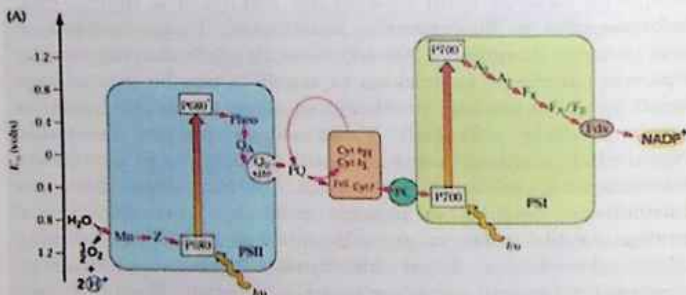
36-rasm. Fotosintezning fototizimi strukturasi
