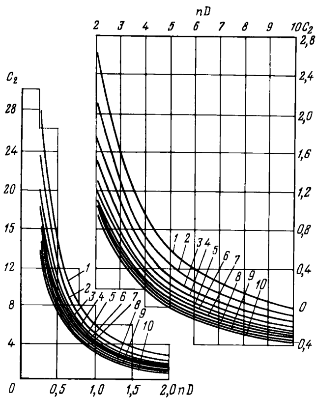
Рис. 4.12. Графики В. И. Щурова для определения коэффициента C_2 при l = 0.5 . Номерам кривых соответствуют значения \alpha : 1–0,02; 2–0,04; 3–0,06; 4–0,08; 5–0,1; 6–0,12; 7–0,14; 8–0,16; 9–0,18; 10–0,2
