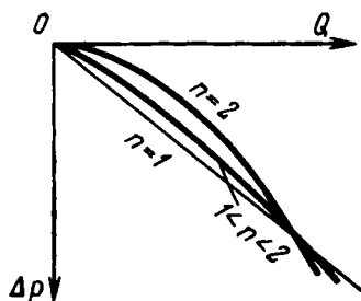
Рис. 3.13. Индикаторные линии, соответствующие различным законам фильтрации жидкости
