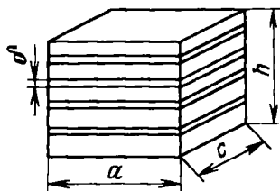
Рис. 12.2. Модель трещиноватой среды с упорядоченной системой трещин
