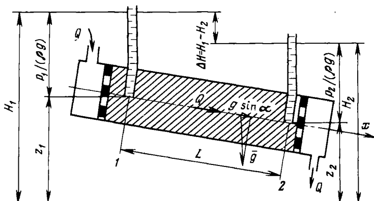
Рис. 1.4. Схема пермеаметра
