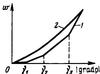
Рис. 11.4. Зависимости скорости фильтрации от модуля градиента давления:
