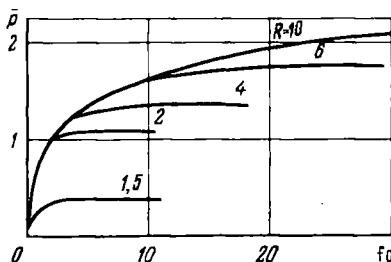
Рис. 5.18. Зависимость безразмерной депрессии \bar{p} от параметра Фурье f_0 для укрупненной скважины, расположенной в открытом пласте конечного размера ( Q_u = \text{const} , R = R_x/R_1 )
