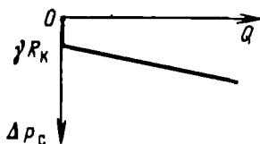
Рис. 11.5. Индикаторная линия при плоскорадиальной фильтрации ВПЖ
