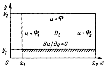
Рис. 13.7. Схема области фильтрации упругой жидкости
