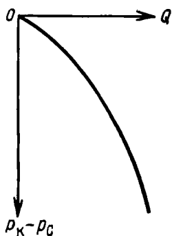
Рис. 3.14. Индикаторная линия при фильтрации жидкости по двучленному закону
