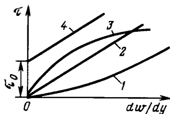
Рис. 11.1. Зависимость касательного напряжения от градиента скорости для различных моделей жидкости:
