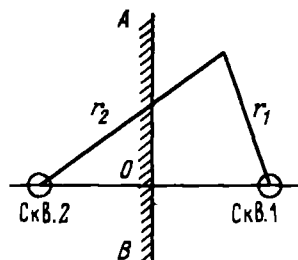
Рис. 5.6. Схема полубесконечного пласта с прямолинейной непроницаемой границей
