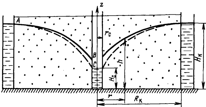
Рис. 3.22. Схема безнапорного притока к совершенной скважине
