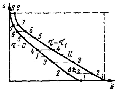
Рис. 9.3. Деформация профиля насыщенности при смешивающемся вытеснении
