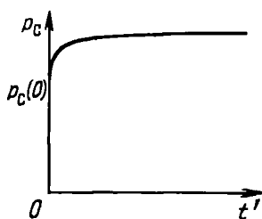
Рис. 6.2. Кривая восстановления забойного давления после остановки скважины
