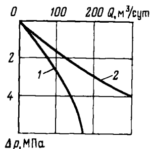
Рис. 12.3. Индикаторная линия для добывающей (1) и нагнетательной (2) скважин в деформируемом трещиноватом пласте
