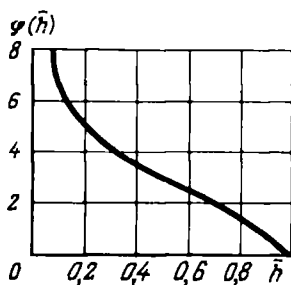
Рис. 4.10. График функции \varphi(\bar{h}) , определенной по формуле (4.25)
