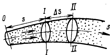
Рис. 2.3. Трубка тока
