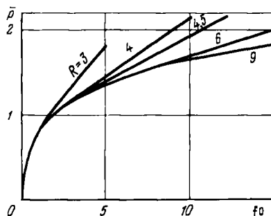
Рис. 5.17. Зависимость безразмерной депрессии \bar{p} от параметра Фурье f_0 для укрупненной скважины, работающей в закрытом пласте конечного размера ( Q_u = \text{const} , R = R_x/R_1 )
