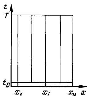
Рис. 13.4. Схема полудискретного аналога непрерывной области фильтрации
