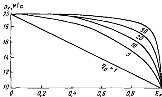
Рис. 7.4. Изменение давления на границе раздела жидкостей ( p_x = 20 МПа, p_r = 10 МПа)
