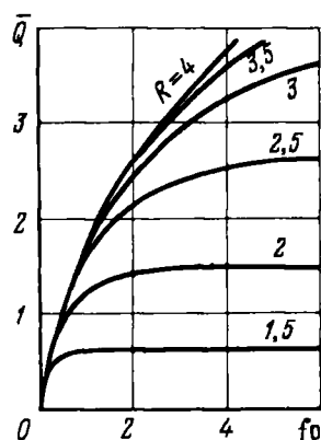
Рис. 5.16. Зависимость безразмерного объема \bar{Q} отобранного из укрупненной скважины, от параметра Фурье f_0 для закрытого пласта конечного размера ( p_e = \text{const} , R = R_x/R_1 )
