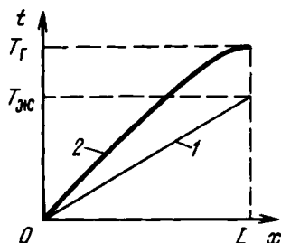
Рис. 3.7. Зависимости t = t(x) частицы в прямолинейно-параллельном потоке:
