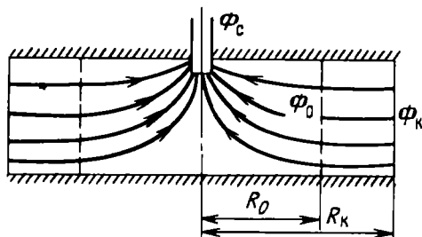
Рис. 4.13. Схема притока к несовершенной скважине, вскрывшей пласт на малую глубину ( b \ll h )
