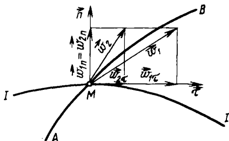
Рис. 7.1. Преломление линий тока на границе раздела жидкостей
