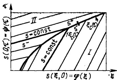
Рис. 9.6. Схема к построению решения обобщенной задачи Бакли-Левверетта
