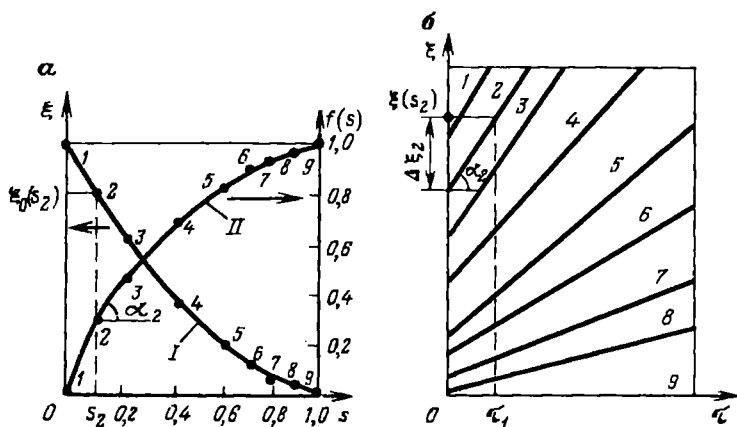
Рис. 9.4. Графическое построение непрерывного профиля насыщенности методом характеристик.
