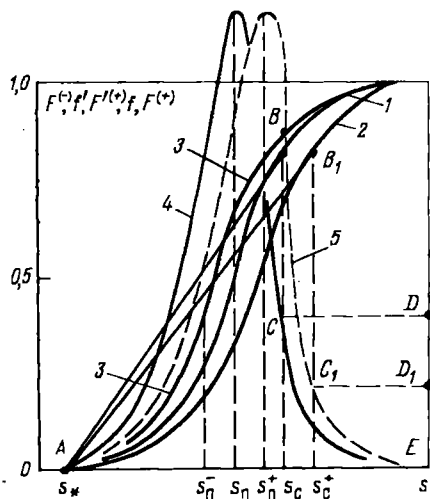
Рис. 9.11. Характеристические функции:
