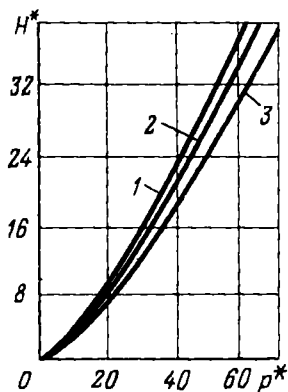
Рис. 9.20. Зависимости безразмерной функции Христиановича от безразмерного давления. а: 1 - 0,02; 2 - 0,015; 3 - 0,01
