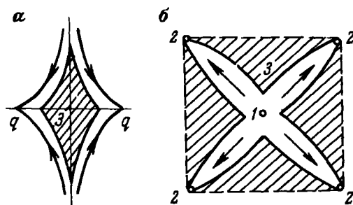
Рис. 11.8. Схема образования застойных зон (3):
