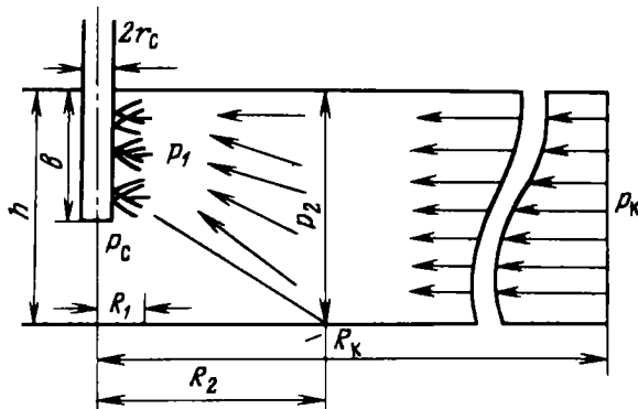
Рис. 4.14. Схема притока газа к неидеальной по степени и характеру вскрытия скважине
