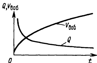
Рис. 5.2. Зависимости дебита и добычи жидкости от времени после пуска галереи при условии p_r = \text{const}
