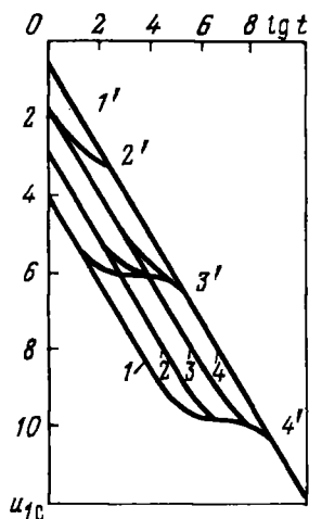
Рис. 12.7. Динамика давления в трещинах на заброс скважины для разных значений параметров \omega и \lambda .
