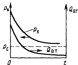
Рис. 6.5. Динамика давления на границе замкнутого газового пласта p_k(t) и дебита Q_{ат}(t) при постоянном забойном давлении
