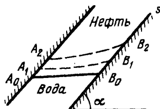
Рис. 7.7. Схема движения водонефтяного контакта в наклонном пласте
