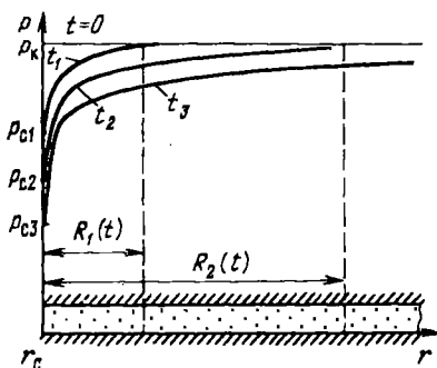
Рис. 5.9. Кривые распределения давления в плоскорадиальном потоке в разные моменты времени по методу ПССС (отбор осуществляется при условии Q = \text{const} )
