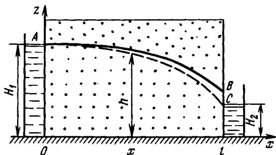
Рис. 3.21. Схема безнапорного течения через прямоугольную перегородку
