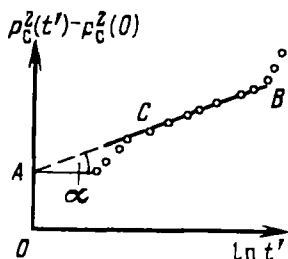
Рис. 6.3. Зависимость p_c^2(t') - p_c^2(0) от \ln t'
