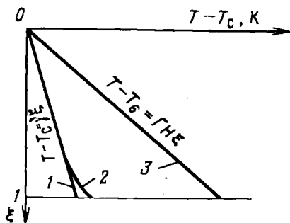
Рис. 10.5. Распределение температуры по глубине залежи:
