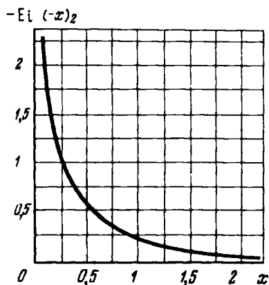
Рис. 5.3. График интегральной показательной функции
