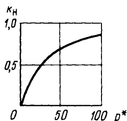
Рис. 9.19. Зависимость относительной фазовой проницаемости от p^*
