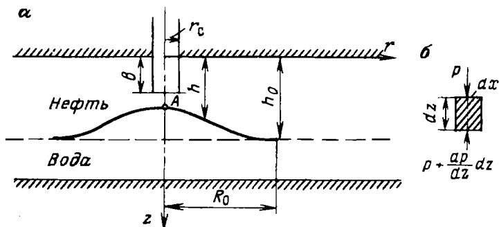
Рис. 7.11. Схема конуса подошвенной воды
