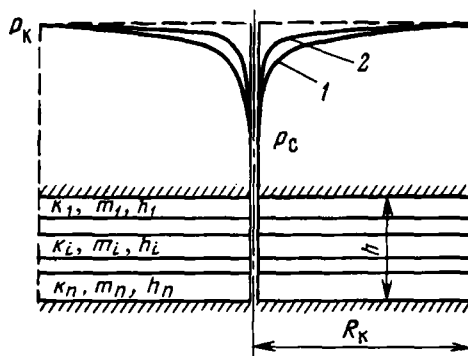
Рис. 3.19. Кривые распределения давления для жидкости (1) и для газа (2) в плоскорадиальном потоке в слоисто-неоднородном пласте
