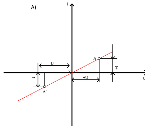
1-rasm: Passiv chiziqli elementlarning volt-ampere xarakteristikasi
