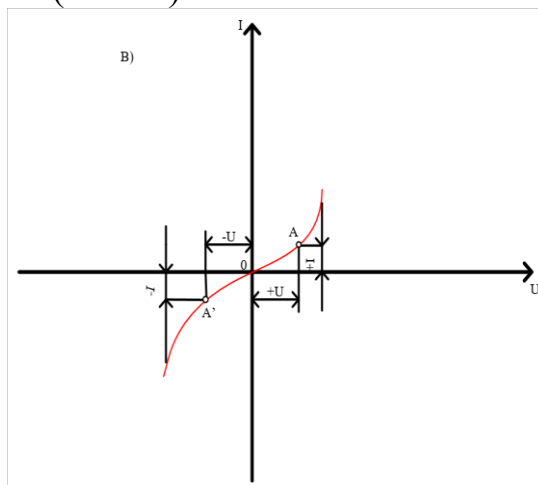
2-rasm: Passiv nochiziqli, simmetrik elementlarning volt-ampere xarakteristikasi
