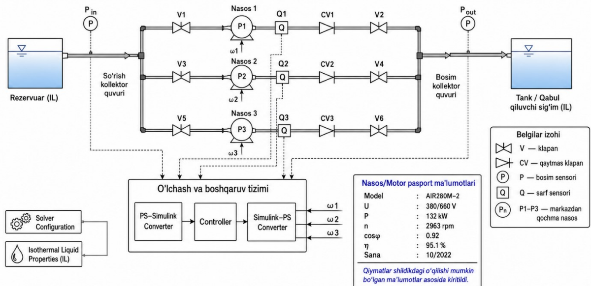
1-rasm. Shaxta suv chiqarish tizimining MATLAB/Simulink muhitida yaratilgan boshqaruv va monitoring elementlari bilan integratsiyalashgan simulyatsion modeli
