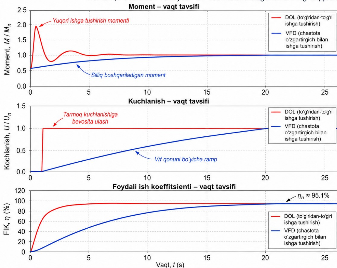
2-rasm. Shaxta suv chiqarish nasosi elektr yuritmasini to‘g‘ridan to‘g‘ri va chastota o‘zgartirgich yordamida boshqarish usullarida ishga tushirish jarayonining moment, kuchlanish va foydali ish koeffitsienti bo‘yicha qiyosiy taxlili
