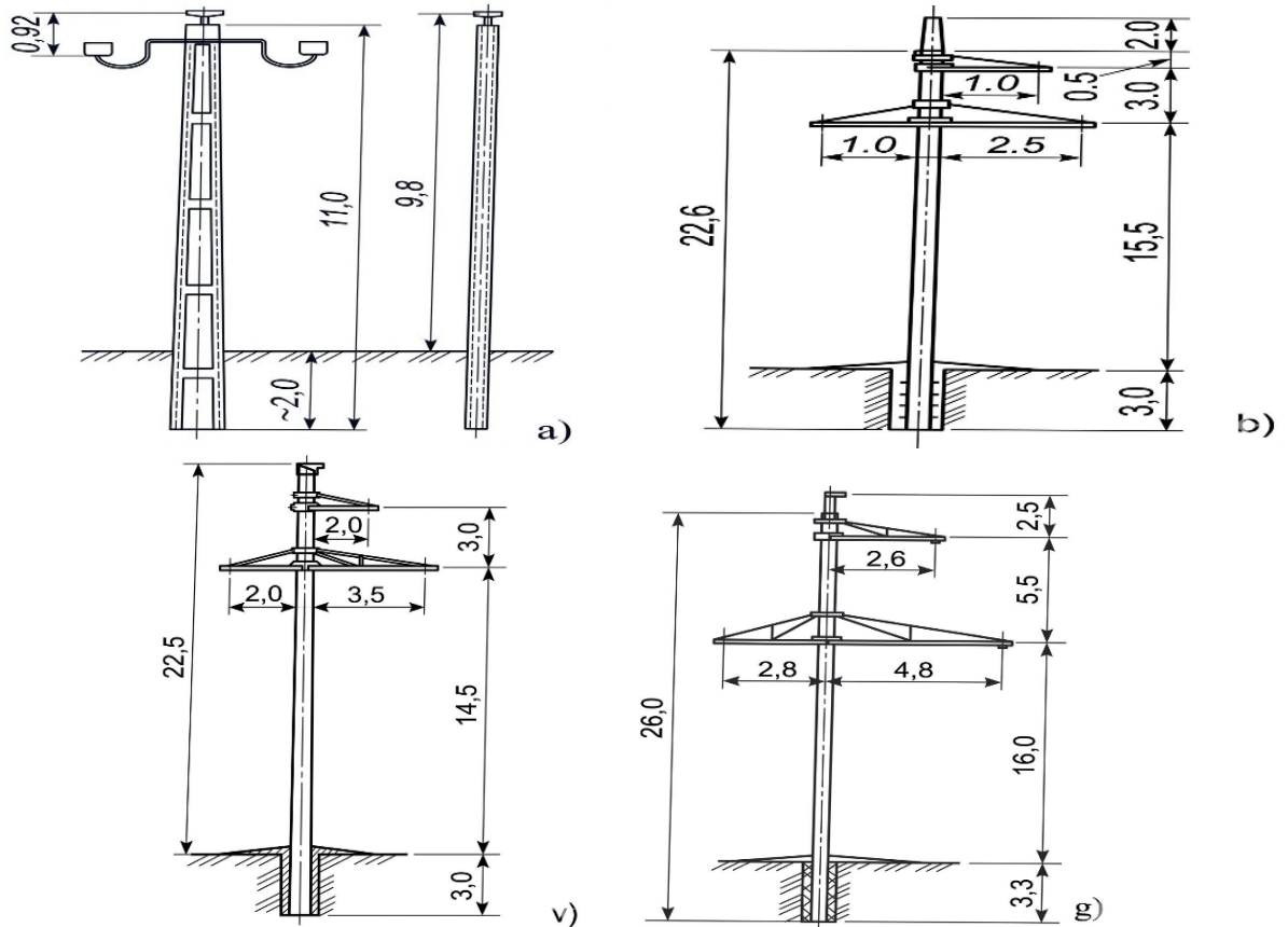
1-rasm. Erkin joylashuvchi temir-beton oraliq tayanchlar a)-6-10 kV (shtirli izolyatorlar bilan) kuchlanishli havo linyalari tayanchi; b) 35kV kuchlanishli havo linyalari tayanchi; v) 110 kV kuchlanishli havo linyalari tayanchi; g) 220 kV kuchlanishli havo linyalari tayanchi
