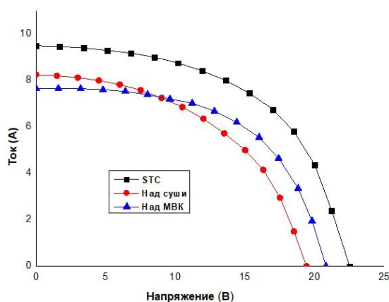
Рис.2. Нагрузочная ВАХ ФЭМ на основе СЭ из поликристаллического кремния мощностью 170 Вт
