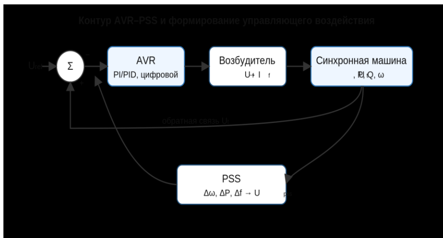
Рисунок 2 – Контур AVR–PSS и формирование управляющего воздействия Стабилизатор энергосистемы PSS
