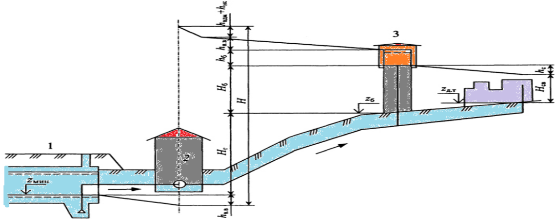
2– rasm. «Bobotog» nasos stansiyasining suv ko‘tarib berish tizimini qirqimi keltirilgan.
