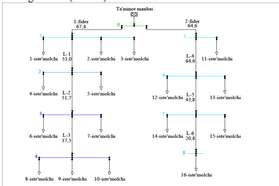
1-rasm. Past kuchlanishli elektr tarmog'ı
