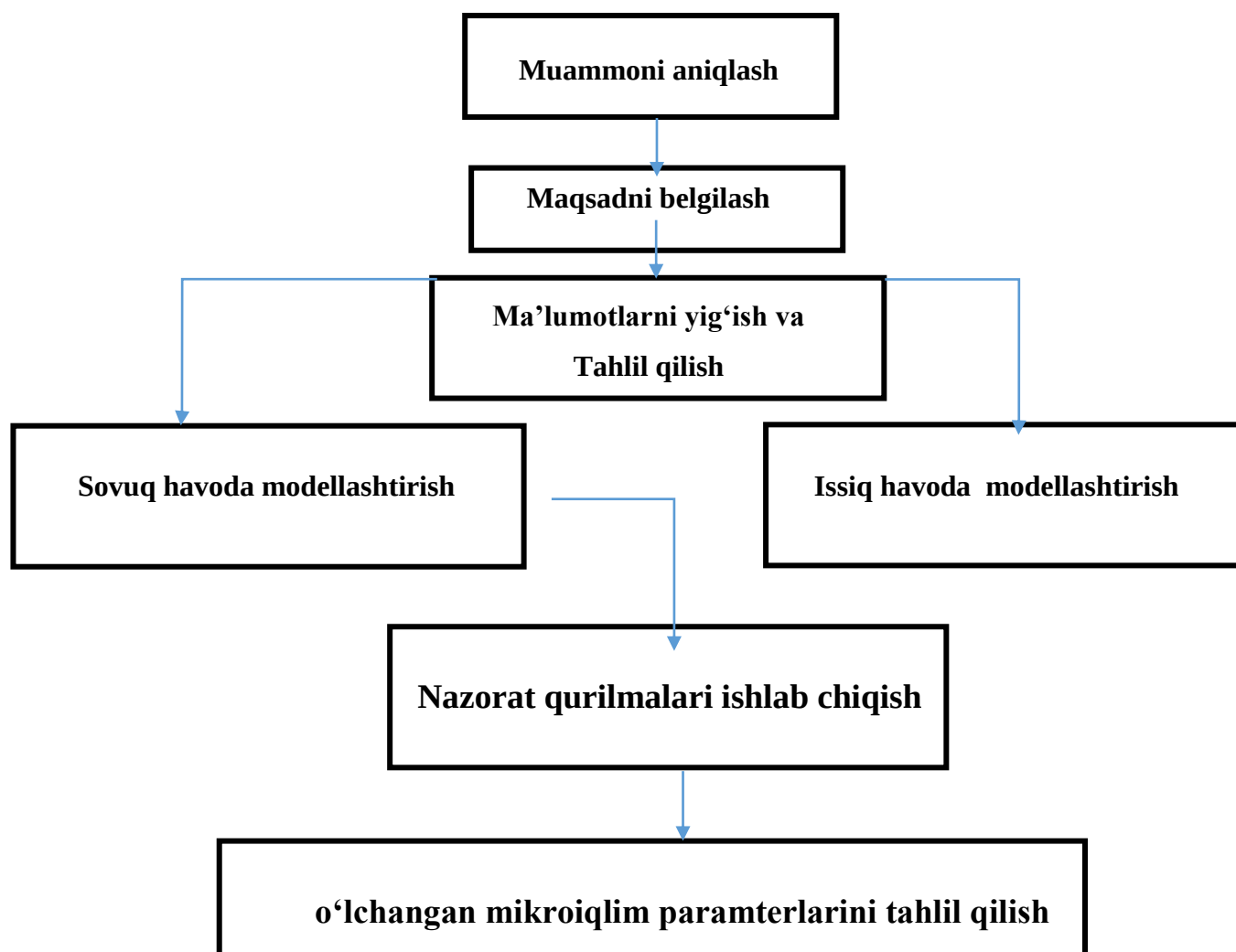
2-rasm. Issiqxona iqlim nazoratini ishlab chiqish algoritmi
