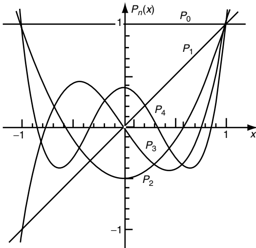
Fig. 4.5. Legendre polynomials
