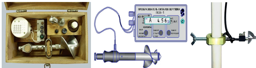
3.3-расм. Сув оқимининг тезлигини ўлчайдиган вертушка
