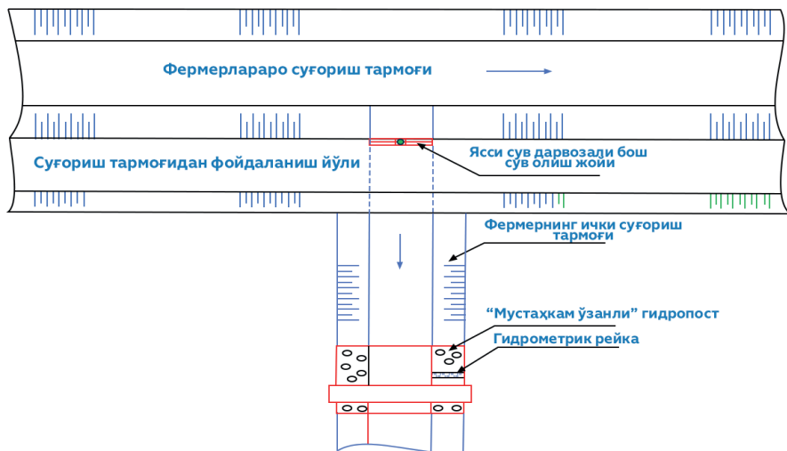
2.1-расм. Очиқ суғориш тармоғидаги сув олиш жойининг схемаси
