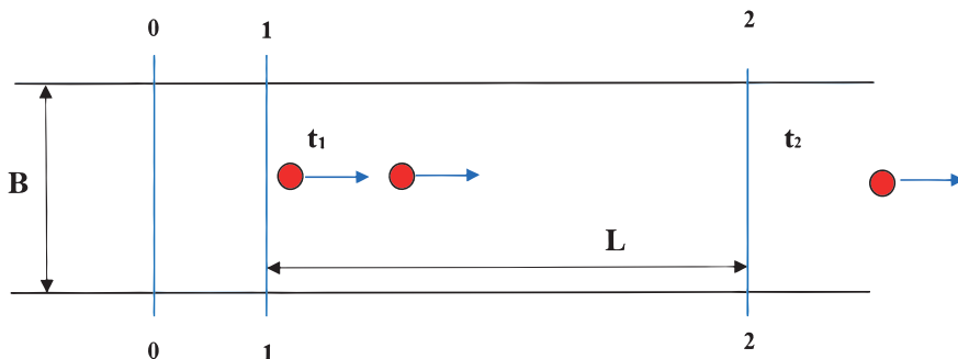
3.2-расм. Сув сарфини “пўкак” ёрдамида ўлчаш
