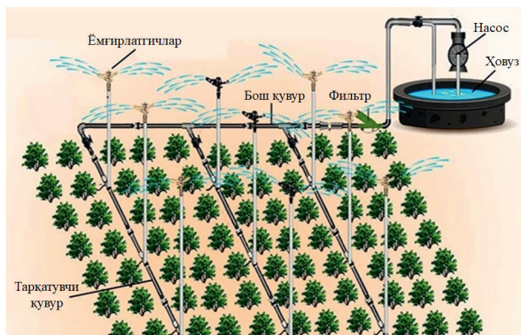
28-расм. “Спринклер” ёмғирлатиш tizimining sxemasi
