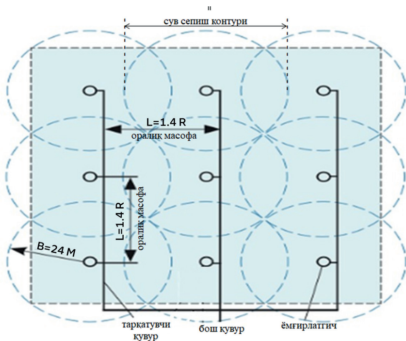
32-расм. Ёмғирлатгичларни сув тарқатувчи қувур бўйлаб ўрнатиш схемаси
