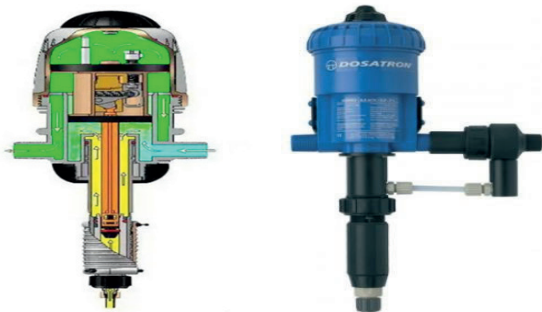
14-расм. Дозатор-насос
