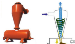
Гидроциклон
