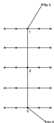
16-расм. Юзани магистраллар усулида нивелирлаш схемаси
