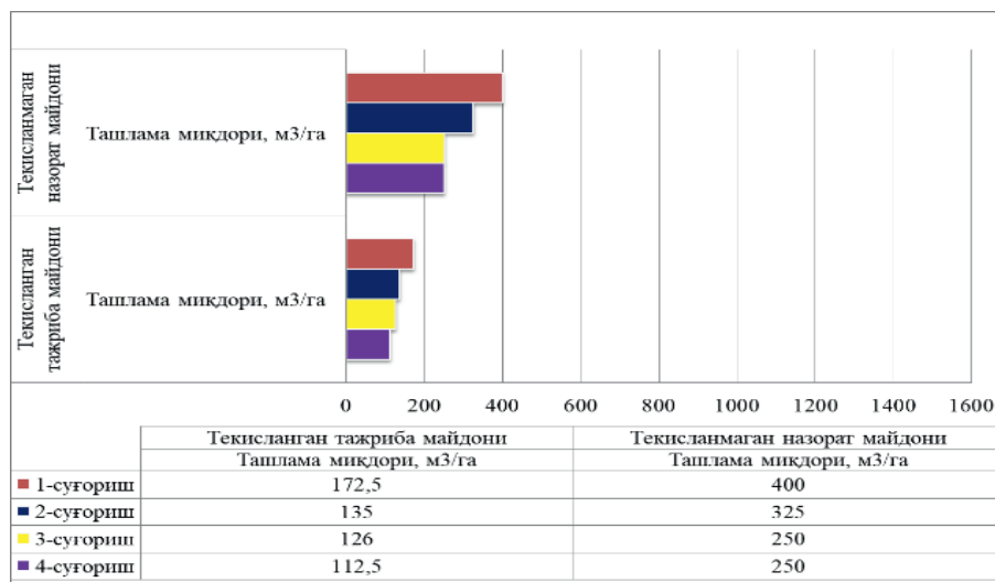
32-расм. Текисланган ва текисланмаган майдонларда кузги бугдойни сўғоришда сўғориш меъёрларининг ва ташлама сувлар миқдорининг ўзгариши
