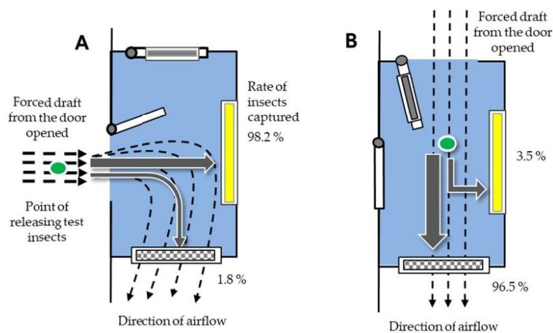
2-rasm. Elektr maydon ekranlari bilan havo oqimiga yo‘naltirilgan anteroomda zararkunandalarni yo‘q qilishning sxematik tasviri
