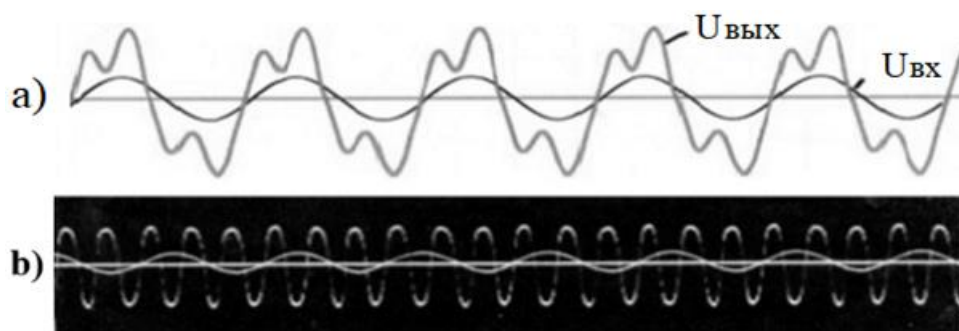
рис.5. Осциллограммы (АОТПЧФич)
