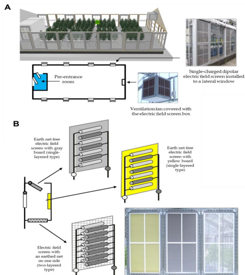
1-rasm. Zararkunandalarni (A) va old xonada (B) o‘rnatilgan uch turdagi elektr maydon ekranlarini butunlay chiqarib tashlaydigan ideal issiqxona.
