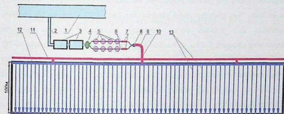
6.8-rasm. Dala tajriba oʻtkazilgan maydon sxemasi.
