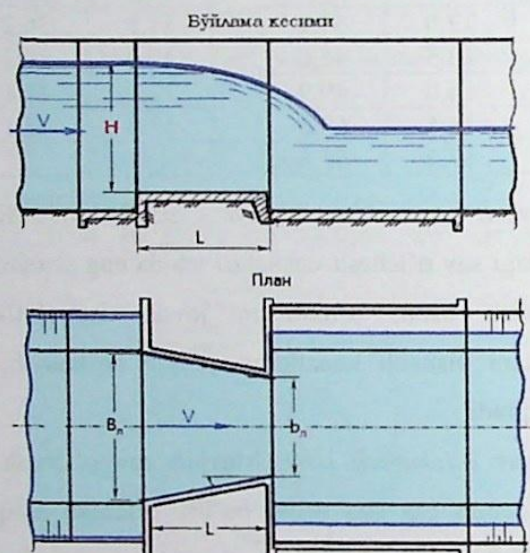
1.5-rasm. SANIIRI suv oʻlchagich novining chizmasi:
