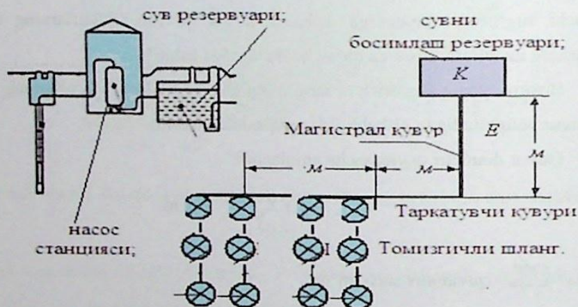
6.20-rasm. Tomchilatib sug'orish tizimining gidravlik sxemasi.
