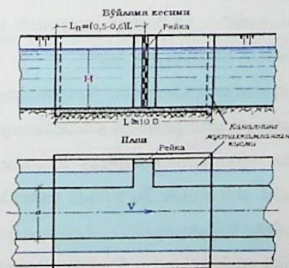
1.7-rasm. O'zgarmas o'zan turidagi suv o'lchash postining chizmasi:
