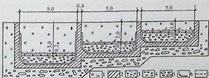
4.4-rasm. Sug'orish texnikasi ilmiy tadqiqod stansiyasining (STITS) Toshkent viloyatidagi lizimetrlar konstruksiyasining sxemasi.
