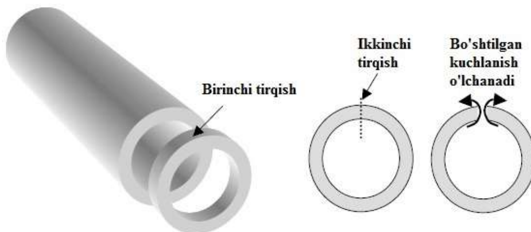
2-rasm: Burovchi momentlaridan qolgan kuchlanishlarni aniqlash uchun filamentli o'ralgan trubalarni kesish.
