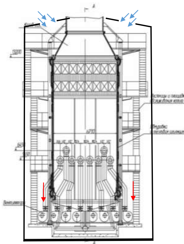
1-рasm: Issiq havo bilan taminlash tizimi.
