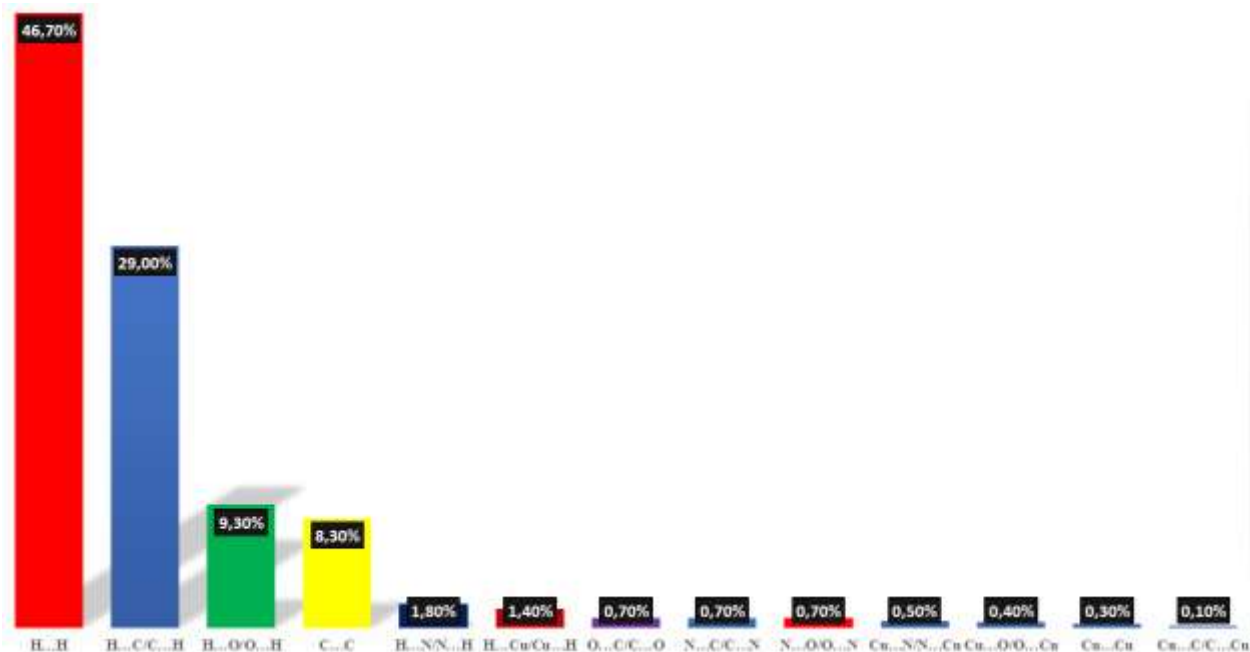
5-rasm. [Cu 24 H 18 O 2 N 2 ] tarkibli kompleksning Hirshfeld barmoq izi diagrammasi
