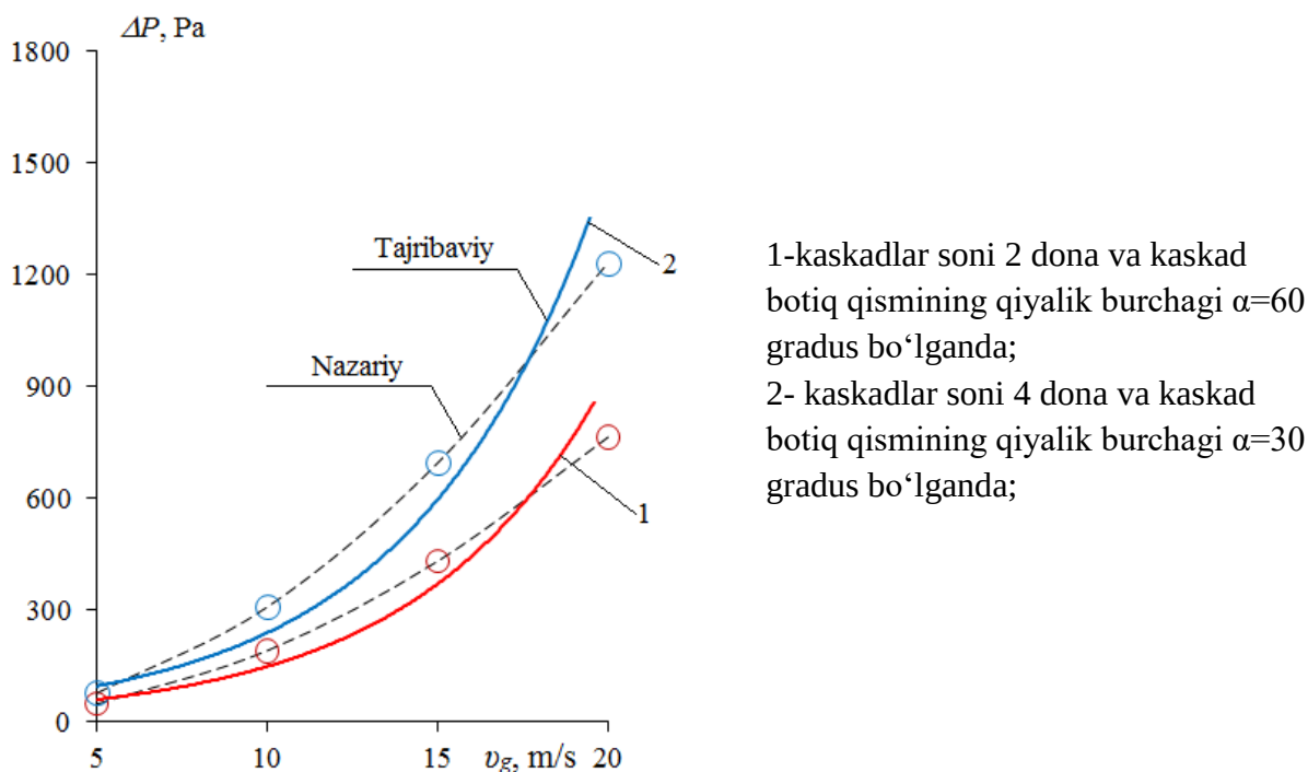
1–rasm. Airadinamik qarshilikning gaz tezligiga bog‘liqligi ( Q_{unm}=0,073 \text{ kg}\cdot\text{s}\cdot\text{const} ).
