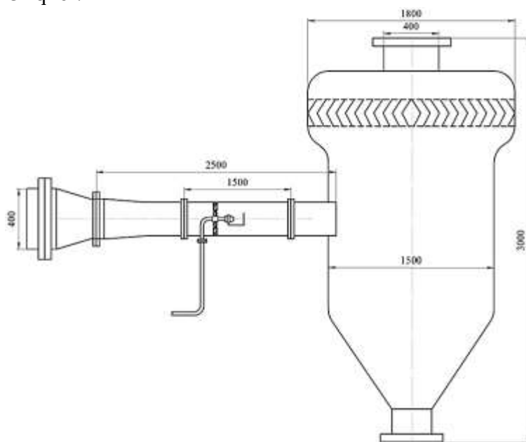
1-rasm. Ho'l usulda chang ushlovchi va gaz tozalovchi apparat umumiy ko'rinishi.
