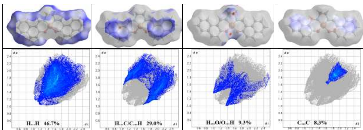
4-rasm. [\text{CuC}_{24}\text{H}_{18}\text{O}_2\text{N}_2] tarkibli kompleks kristallida o'zaro H...H, H...C/C...H, H...O/O...H va C...C ta'sirlashuvlarni ifodalovchi d_{\text{norm}} bo'yicha xaritalangan uch o'lchamli Hirshfeld yuzasi hamda ikki o'lchovli barmoq izlari maydoni
