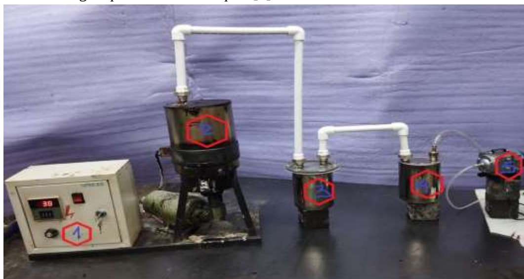
1-rasm. Oltingugurtni modifikatsiya qiluvchi takomillashgan qurilma.
