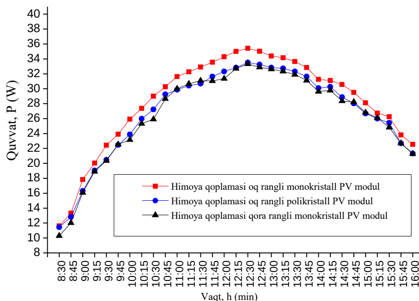
2-rasm. PV modullarning quvvatining vaqt bilan bog'liqligi
