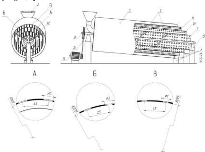
1-rasm. Ko‘p qatlamli barabanli saralash mashinasi.
