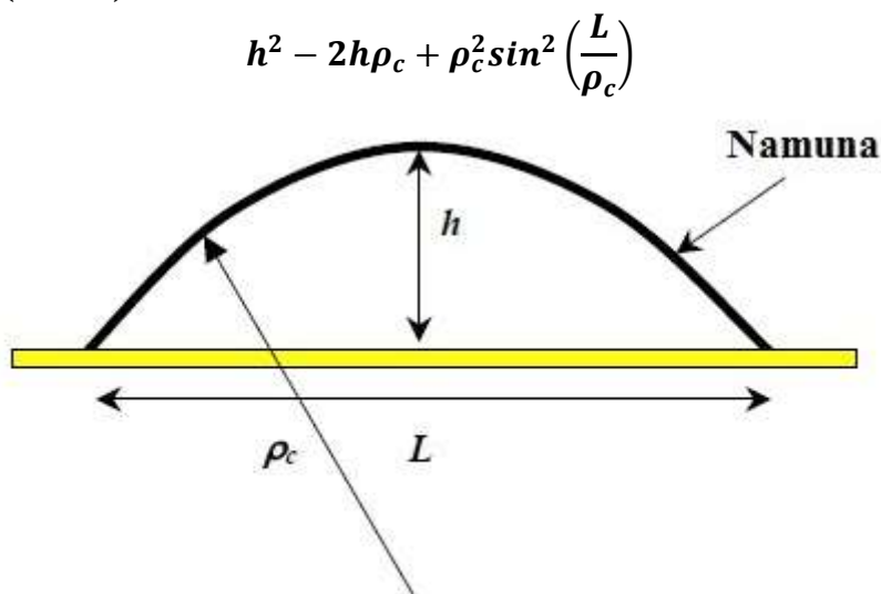
1-rasm: Kompozit chiziqdagi egrilikni aniqlash.
