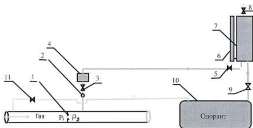
6. Расм – 1. Табиий газга одорат қўшиб бериш схемаси.
