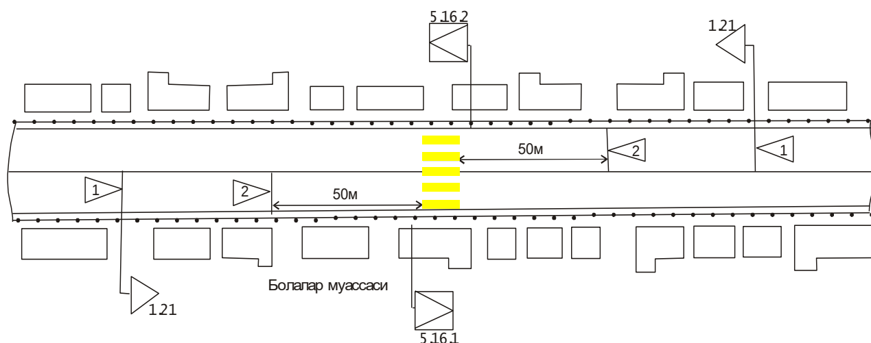
6.17-rasm. Aholi punktidan o'tgan yo'llarda «Piyodalar o'tish joyi» va «Bolalar» yo'l belgi chizig'ini joylashtirish sxemasi.
