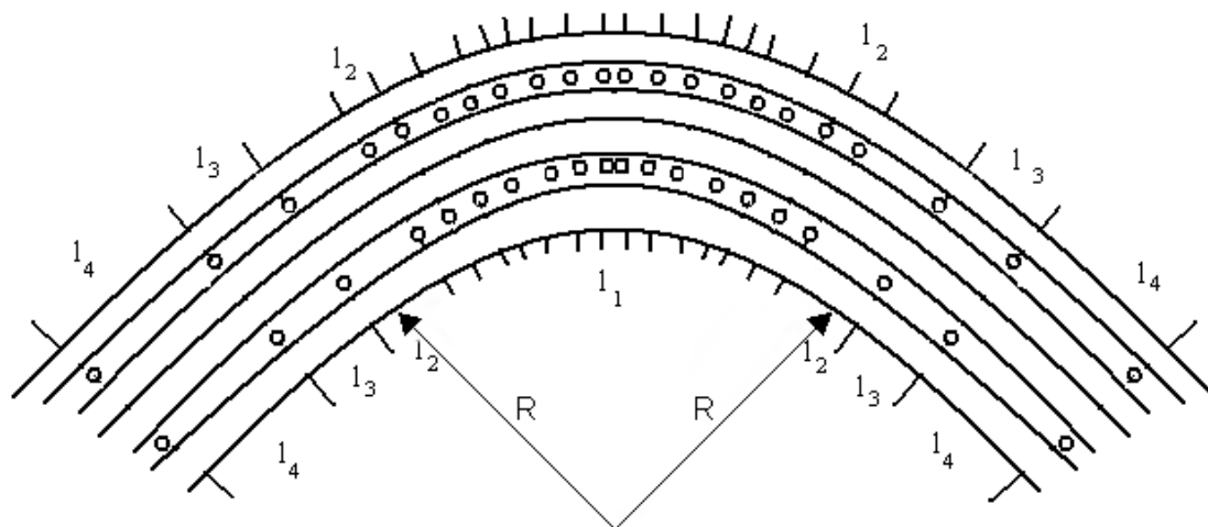
5.13-rasm. Rejadagi egrilikda yo'naltiruvchi ustunchalarni joylashtirish.
