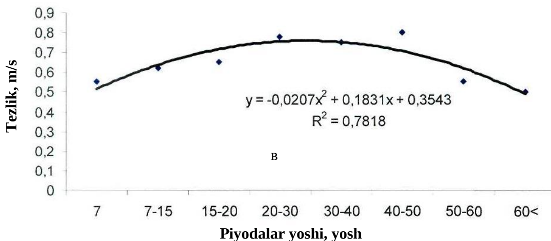
2.9-rasm. Toshkent shahar Amir Temur ko'chasi bo'ylab piyodalarning o'rtacha harakat tezligini o'zgarishi.
