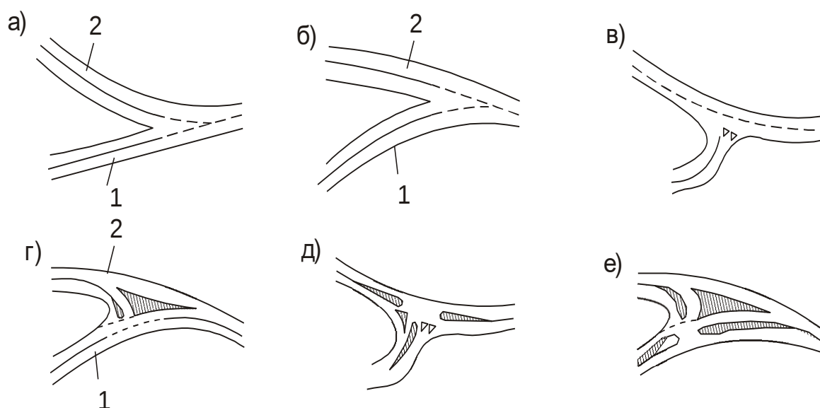
6.3-rasm. Bir sathda tutashishning tavsiya etilgan planirovkasi:
