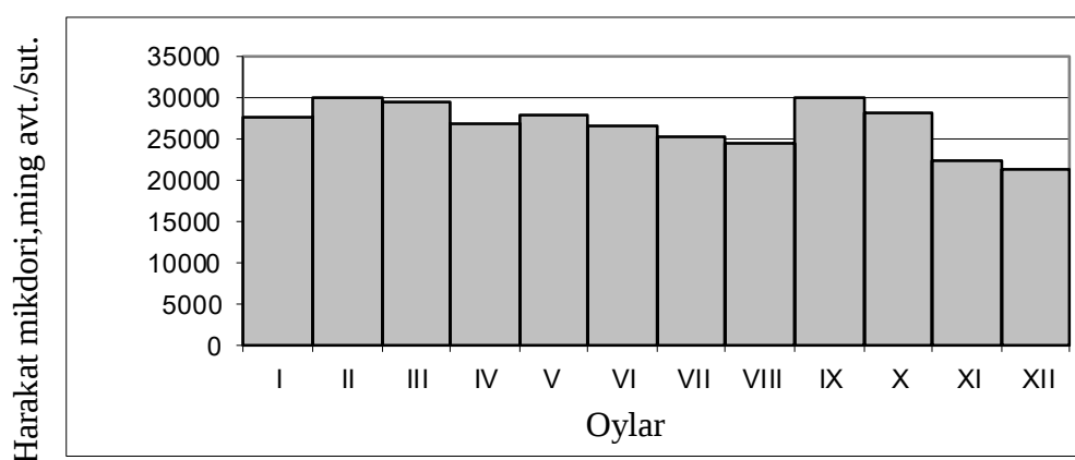
2.2-rasm. Harakat miqdorining oylar bo'yicha o'zgarishi: Amir Temur shox ko'chasi.
