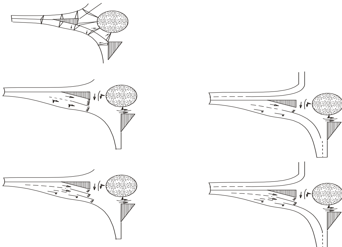
6.7-rasm. Aylanma harakatli chorrahaning chiqish joyini bosqichma-bosqich yaxshilash sxemasi.
