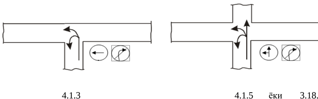
5.7-rasm. Buyuruvchi belgilar bilan o'ng tomonga burilishni ta'qiqlash.
