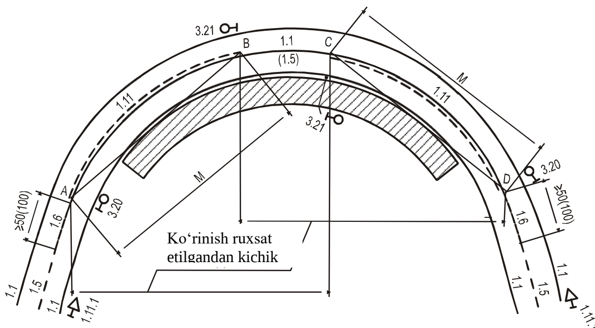
6.11-rasm. Ikki tasmali yo'lining egri bo'lagida ko'rinish ta'minlanmagan holat uchun harakatni tashkil etish sxemasi.
