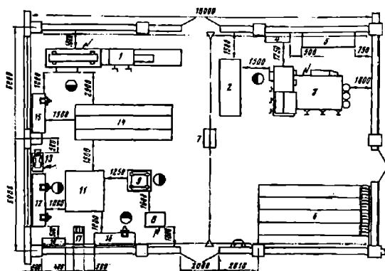
12.6-rasm. Gidroagregatlarni ta'mirlash bo'limining namunaviy ko'rinishi:
