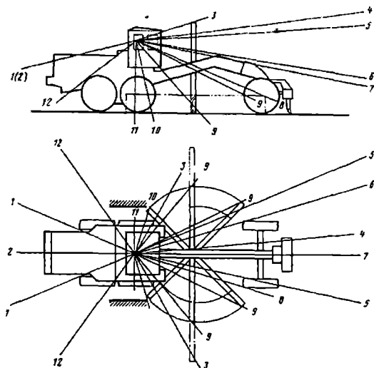
1.3-rasm. Avgreyderlarni boshqarishda ko'rinish jadvali (ВНИИ стройдормаш ma'lumotilari bo'yicha): 1...12 – operatorning ko'rish nurlari.
