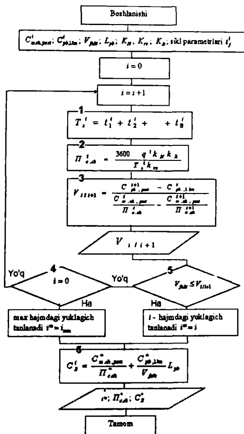
2.1-rasm. OISni belgilovchi algoritmi va bir cho'michli yuk ortkichlarning mos hajmini tanlashning blok tizimi.
