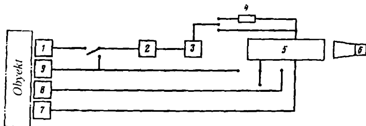
16.7-rasm. Titrash-akustika stendi blok-sxeması.
